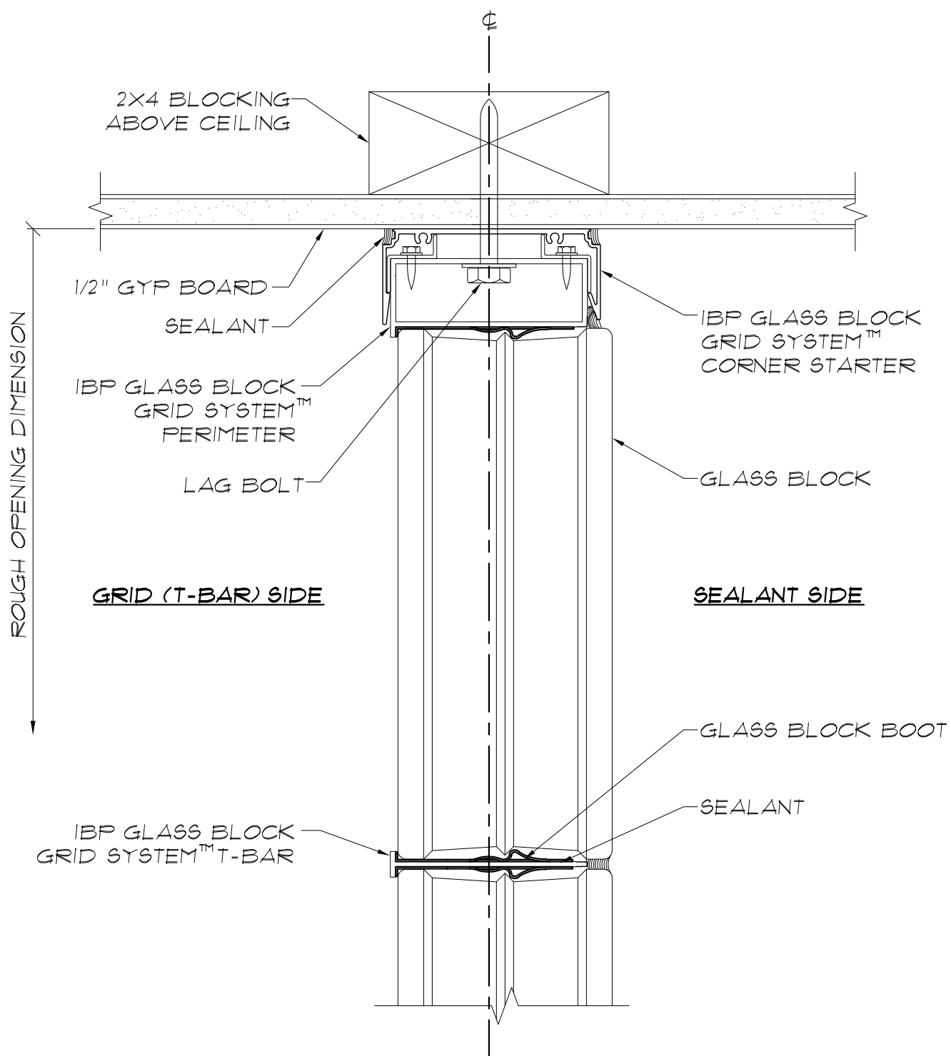
INTERIOR PARTITION AT CEILING SCALE: N.T.S.
