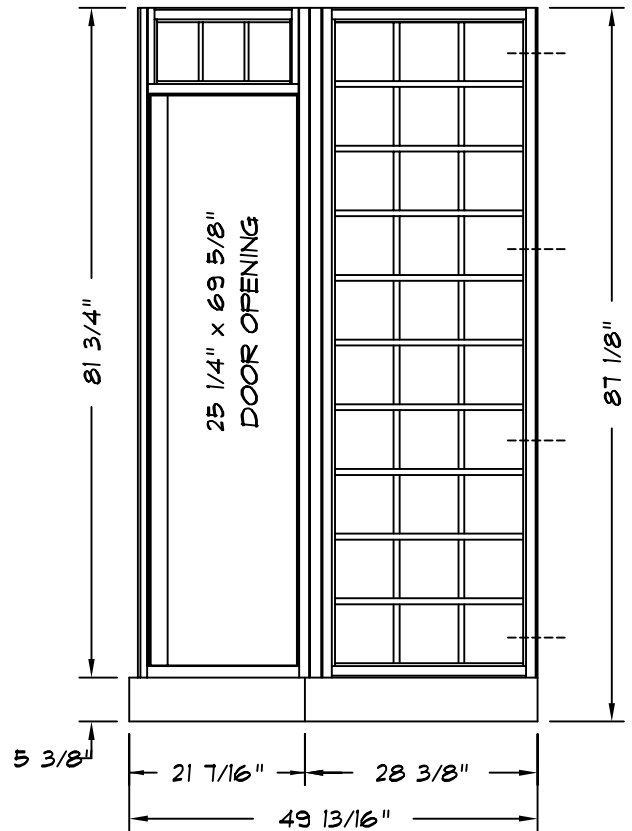
ELEVATION B
