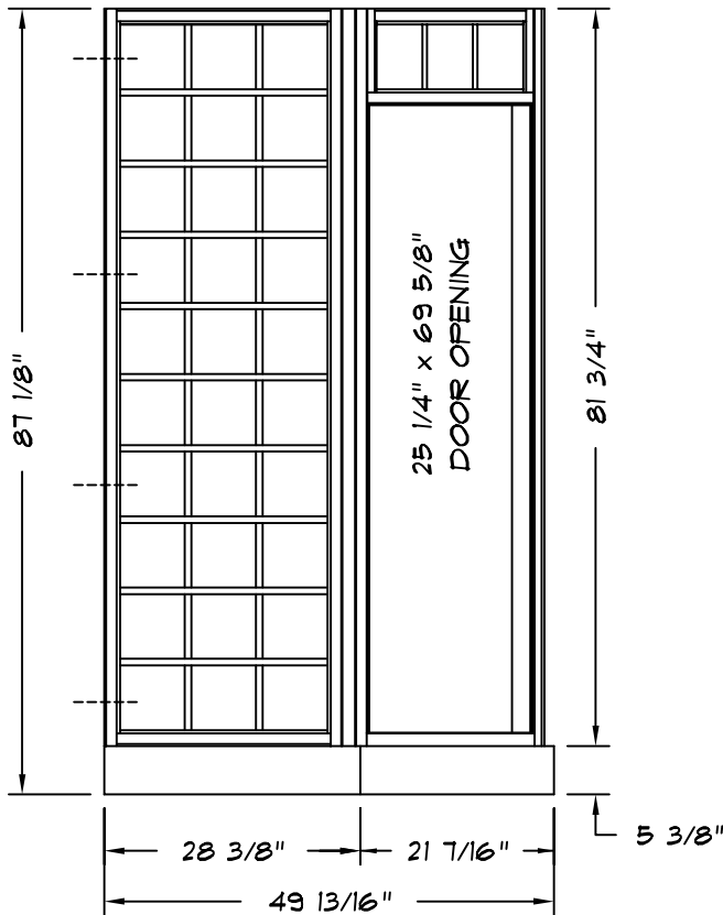
ELEVATION A
