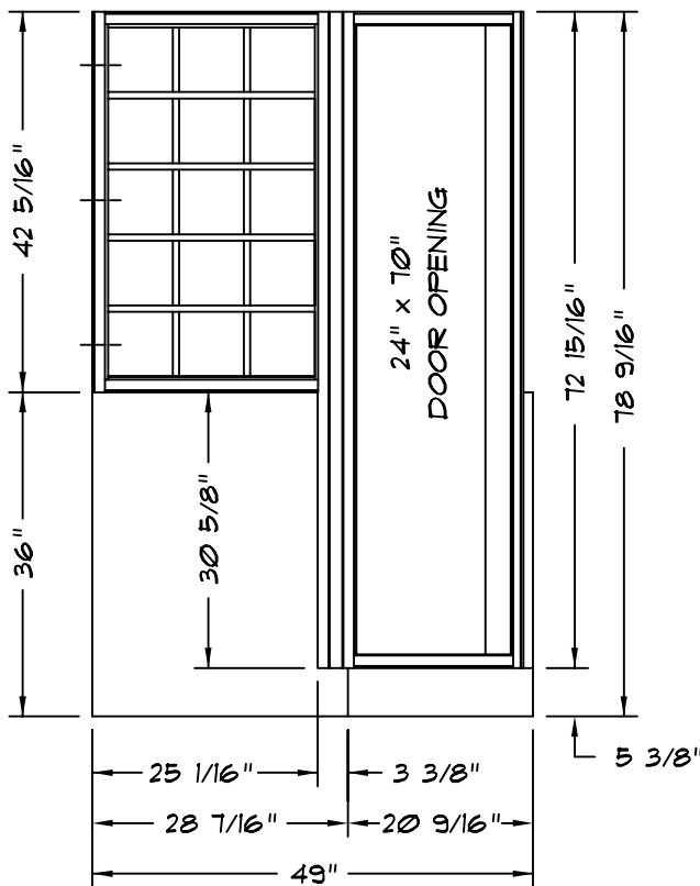
ELEVATION A
