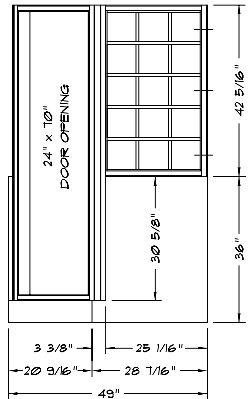
ELEVATION B
