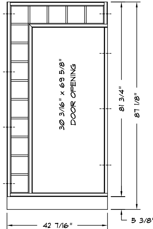
ELEVATION
