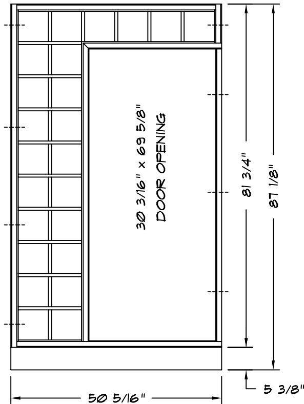
ELEVATION
