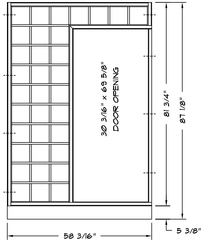
ELEVATION
