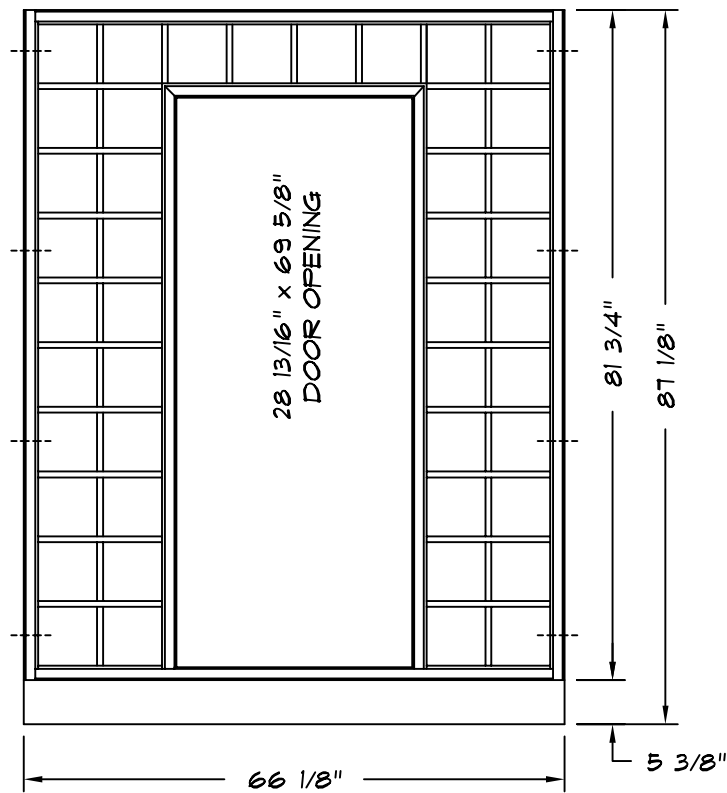
ELEVATION
